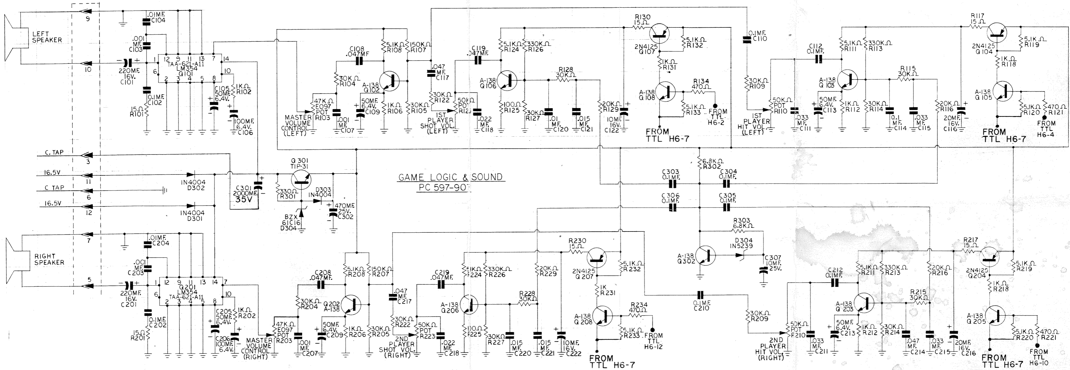
GUN FIGHT SOUND GENERATOR DETAIL P.C. 597-907E
